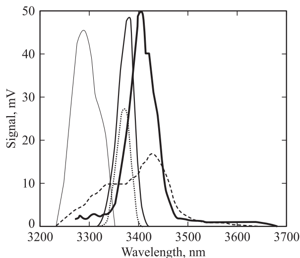
Рис. 2. Спектральный состав излучения образцов \text{Cd}_x\text{Hg}_{1-x}\text{Te} : зависимость интенсивности излучения от длины волны. Различные кривые — различные излучатели из одной пленки \text{Cd}_x\text{Hg}_{1-x}\text{Te} (образец МСТ 638/1, x \approx 0.376 ).
