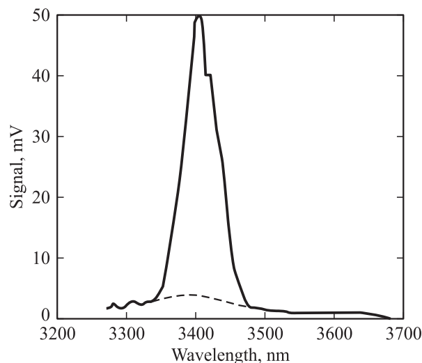
Рис. 1. Спектральный состав излучения образца \text{Cd}_x\text{Hg}_{1-x}\text{Te} при T \approx 77\text{ К} (образец МСТ 638/1, x = 0.376 ). Фотоприемник — образец МСТ 641/1, x \approx 0.272 . Штриховая линия — спектр при интенсивности фотовозбуждения меньше пороговой величины ( P < 4\text{ кВт/см}^2 ). При интенсивностях фотонакачки P \geq 4\text{ кВт/см}^2 на фоне этого пьедестала проявляется узкая линия, изображенная на рисунке сплошной линией.
