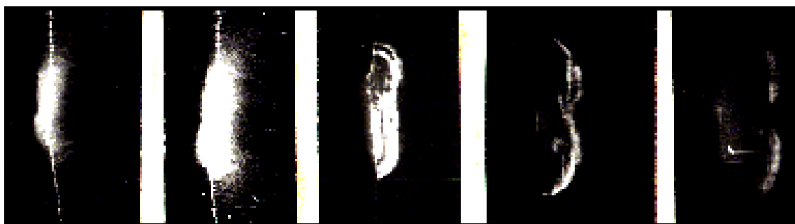
Рис.3. Динамика расширения плазменного микрошнура. Излучающий разряд в воздухе, разрядный промежуток d \approx 0,5 мм, аperiodический импульс тока с амплитудой 750 А имел длительность 400 нс. Экспозиция – 10 нс, интервал между кадрами – 100 нс.
