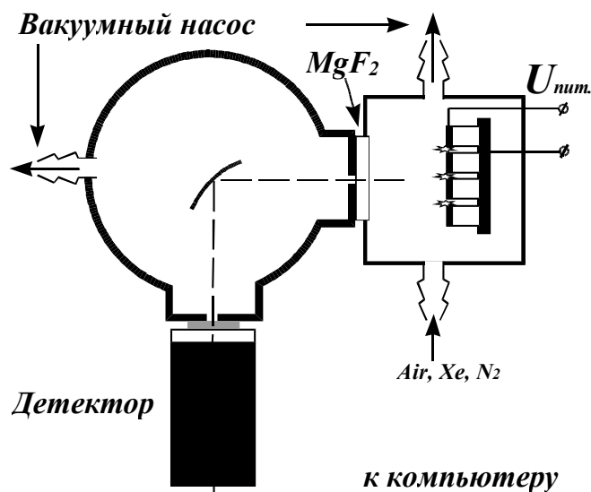
Рис.5. Стенд для исследования спектральных характеристик микроразряда.
