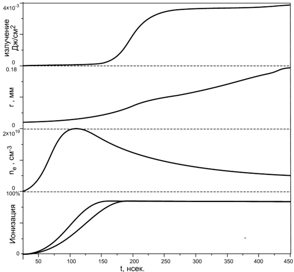
Рис.8. Результаты расчета интенсивности излучения I , радиуса плазменного канала r_0 , концентрации электронов n_e и степени ионизации \zeta от времени разряда t .
