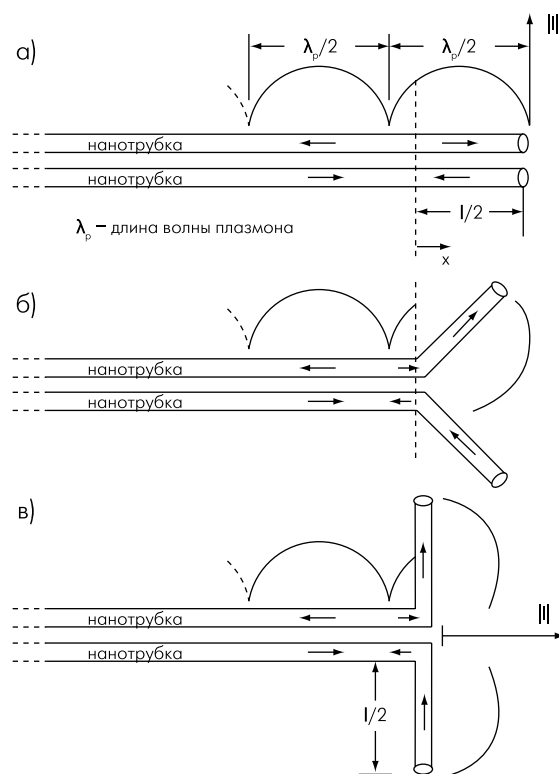
Рис.6. Последовательные стадии трансформации двухпроводной нанопроводной передачи в дипольную наноантенну
