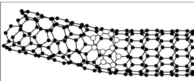
Рис.3. Нанотрубка с внедренным в нее дефектом "семиугольник-пятиугольник" приводит к изгибу трубки и возникновению перехода типа "металл-полупроводник" [11]
